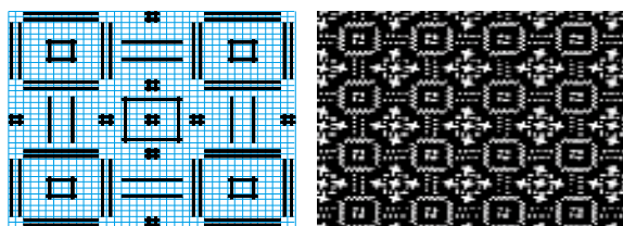
図1 織組織分解図
