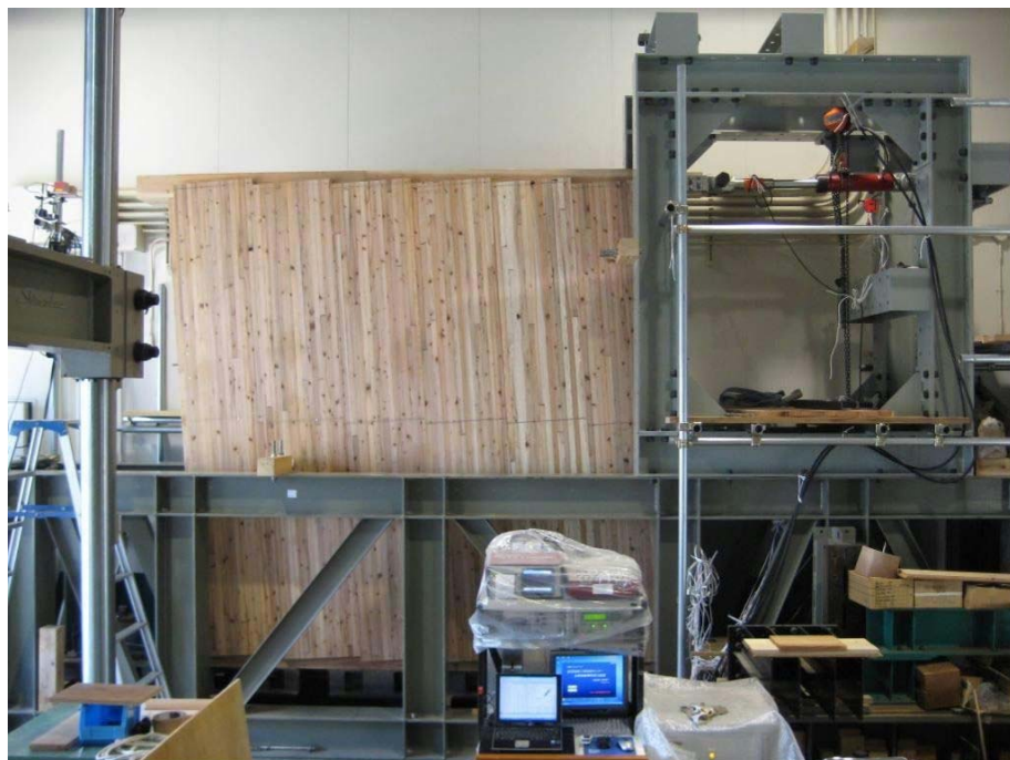
スギ積層パネルを用いた床構面の面内せん断試験
