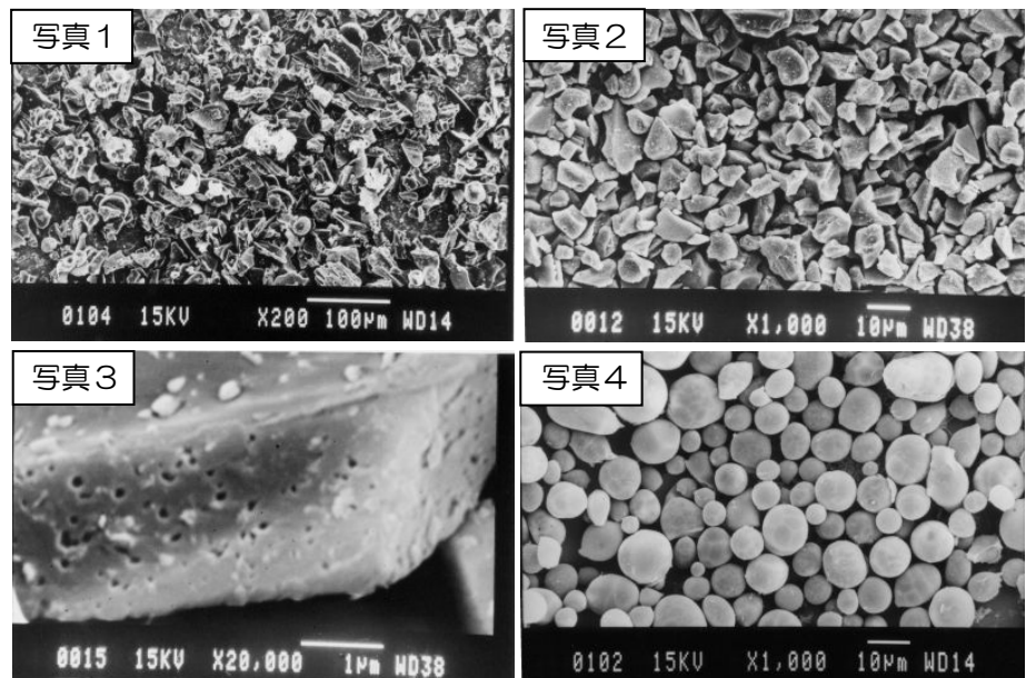
いろいろな形状のシリカの電子顕微鏡写真
