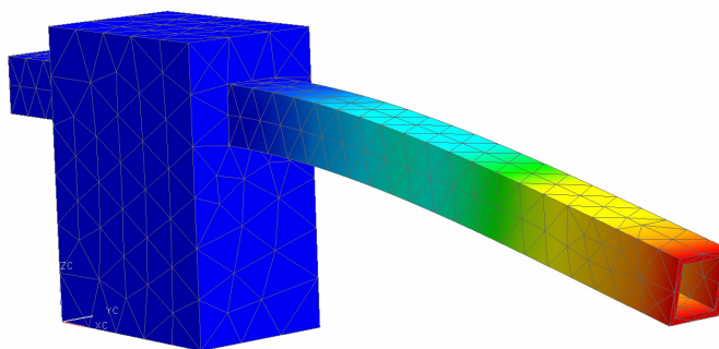
CAEによる構造解析シミュレーション
