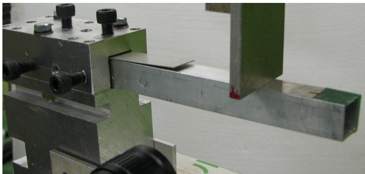
試験機による荷重試験
