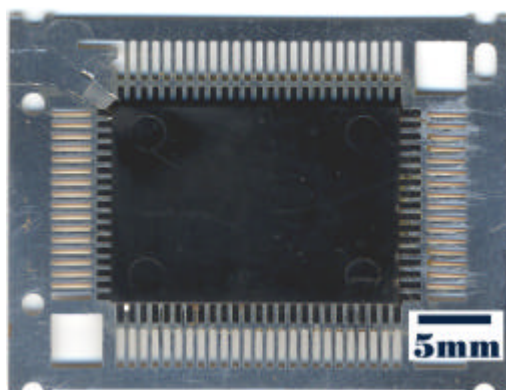
IC 外観写真
