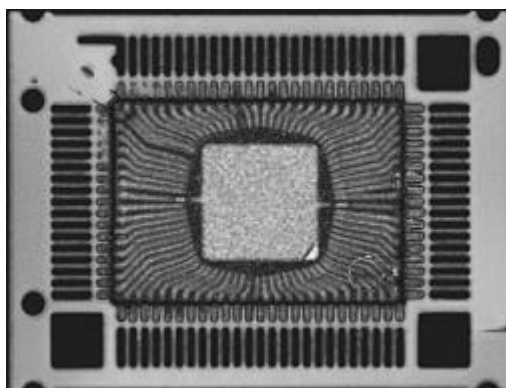
IC パッケージ内部映像
