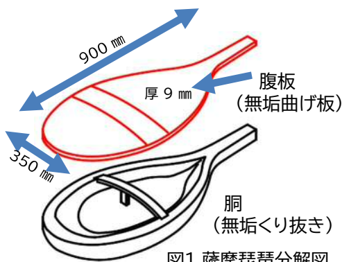
図1 薩摩琵琶分解図
