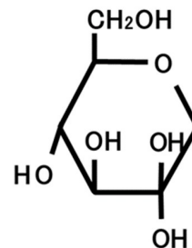
1,5-AFの構造
